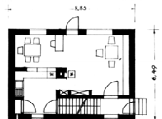
ERDGESCHOSS
