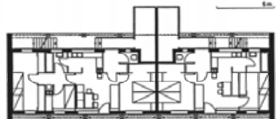
Grundriß des Einfamilien-Doppelwohnhauses.
